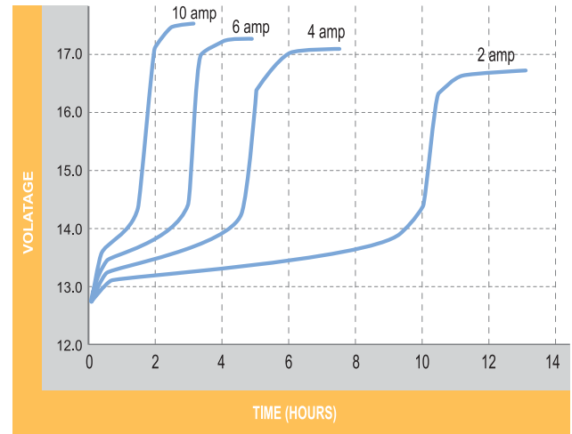
SB 1000 충전특성 (방전심도 20%)
