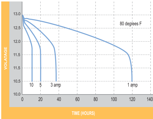
SB 1000 방전특성
